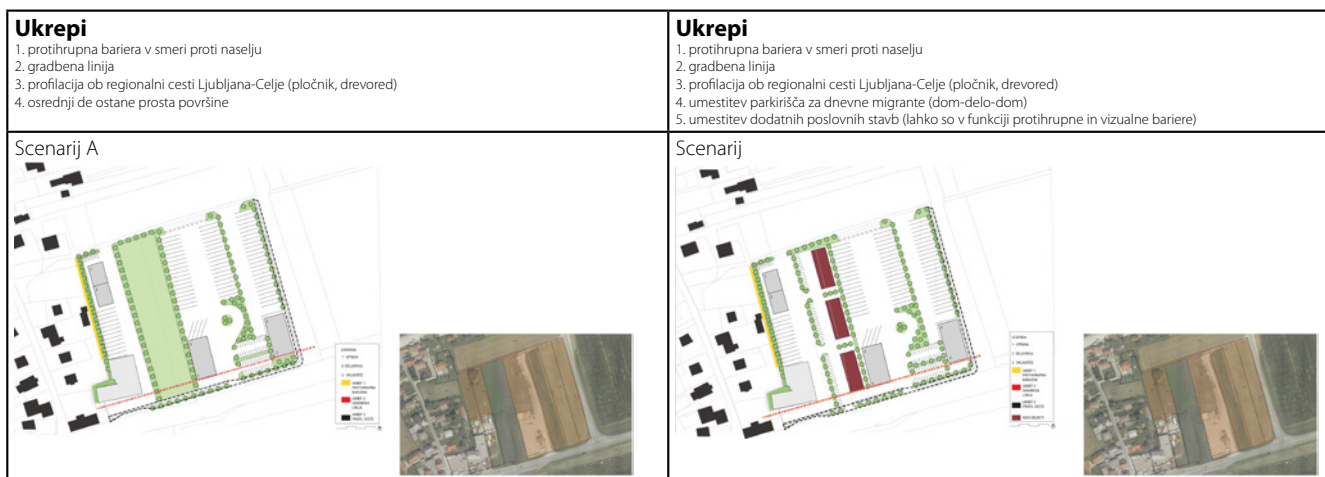
Slika 3: Variantne rešitve zasnove parkirišča in servisnih objektov na lokaciji Šentrupert. Izpostavljeni so posamezni ukrepi za sanacijo hrupa in vizualnega vpliva na naselje.
